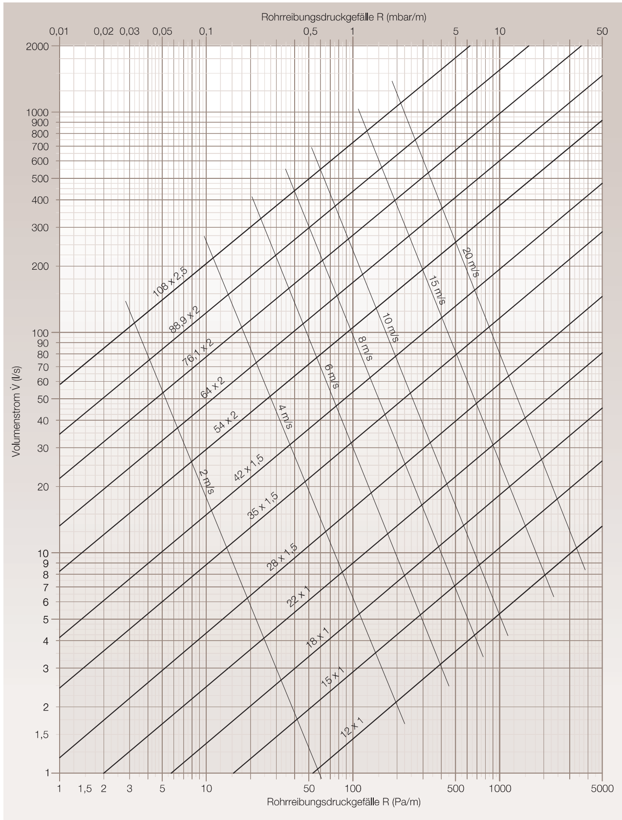
Bild 20. Bestimmung der Druckverluste durch Rohrreibung für Druckluft bei 6 bar Betriebsüberdruck
